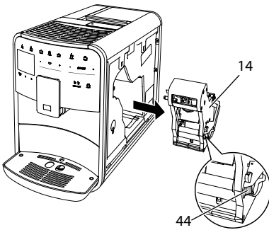
Bild 21: Demontera bryggenheten, 2
