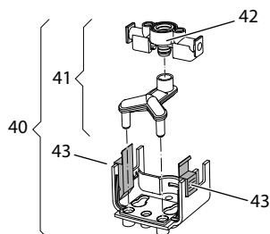
Bild 24: Demontera mjölkenheten, 2
