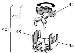
Fig. 19: Dreie innløp, 2
