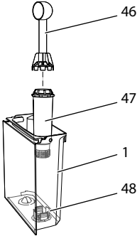
Fig. 25: Enroscar/denroscar el filtro de agua
