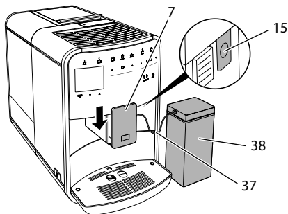
Ilustr. 13: Podłączenie pojemnika na mleko do urządzenia (ilustracja może być odmienną)
